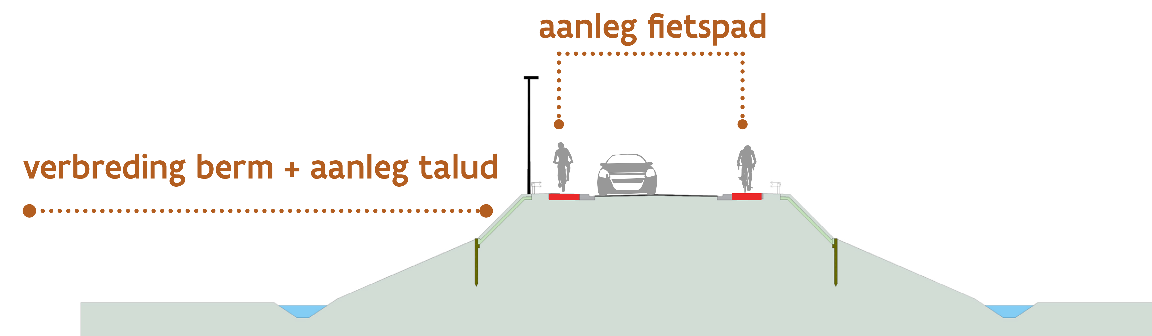
NIEUWE INRICHTING VAN DE AANLOOPHELLING
